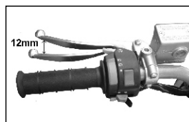
Páka zadní brzdy
